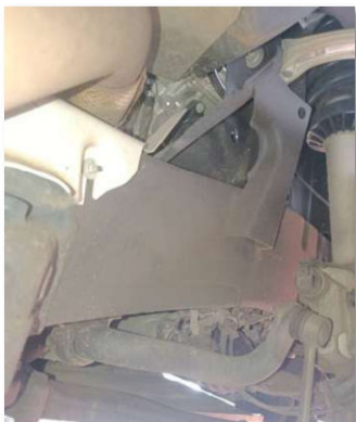
LONGARINA DIANTEIRA DIREITA COM CAIXA DE RODA
