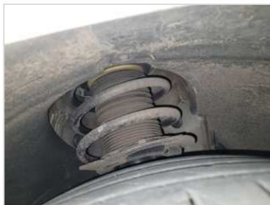
CAIXADE RODADIANTEIRADIREITA
