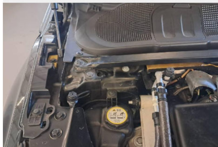
TORRE DO AMORTECEDOR LD
