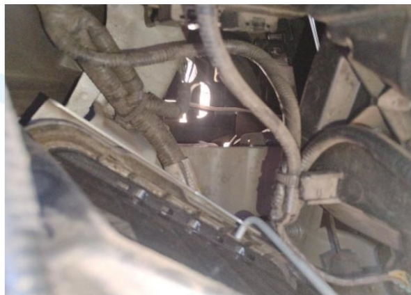
LONGARINA TRASEIRA DIREITA
