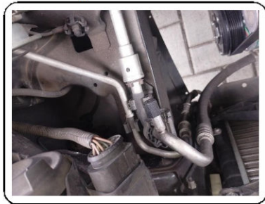
Torre do Amortecedor Direito
