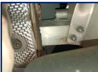
Longarina traseira/esquerda
