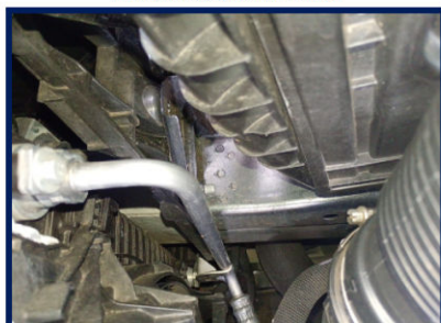
Longarina dianti/direita
