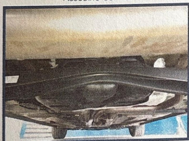
Longarina traseira/direita
