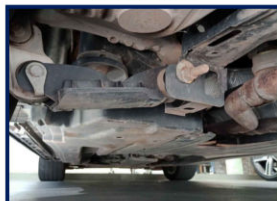
Longarina traseira/direita
