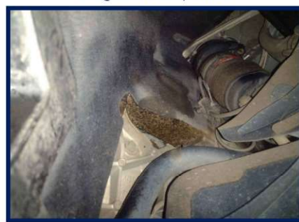
Longarina dianti/direita
